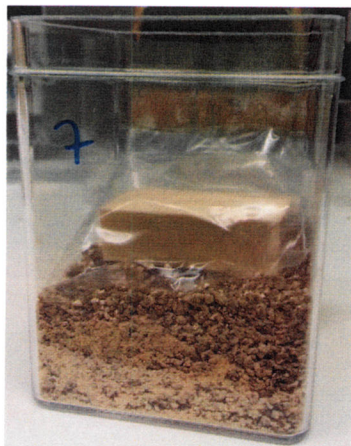
Abb. 02: Platzierung der Materialprobe (Holz in LDPE Folie) im Prüfgefäß (links) mit anschließender Eingrabung in das Substrat (rechts).
